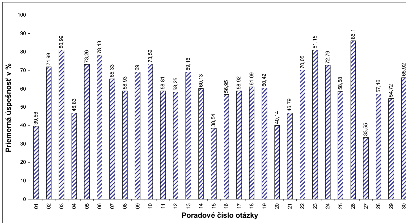
Graf 2 – Obtťažnosť úloh v teste z matematiky v slovenskom jazyku
